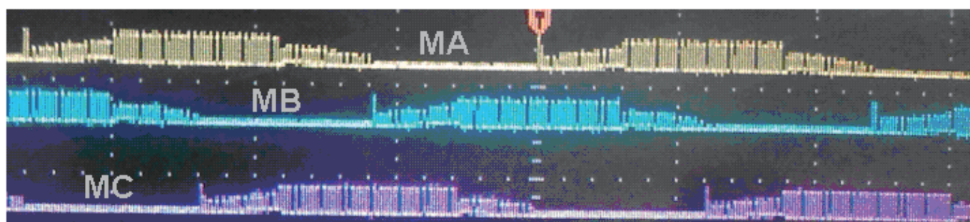
反向驱动输出波形图 (SPWM输出接近正弦波很好的抑制电磁噪音)
